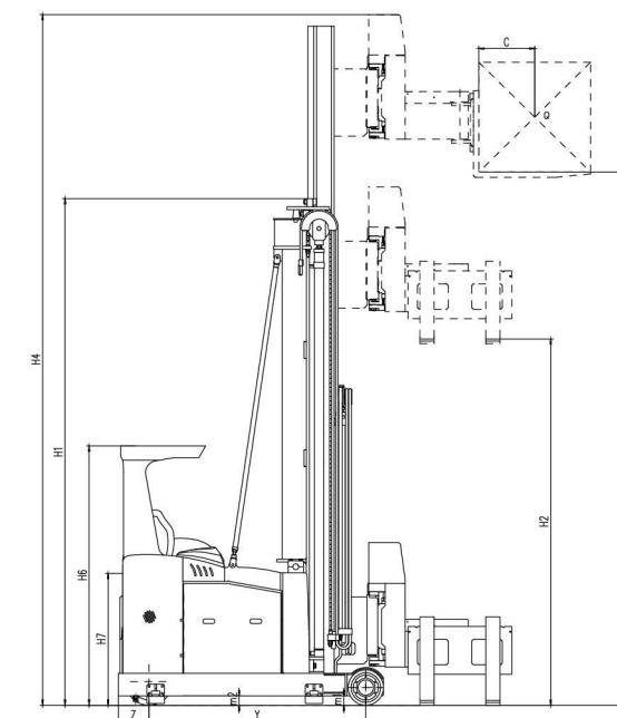
OPD15 Dimensions
